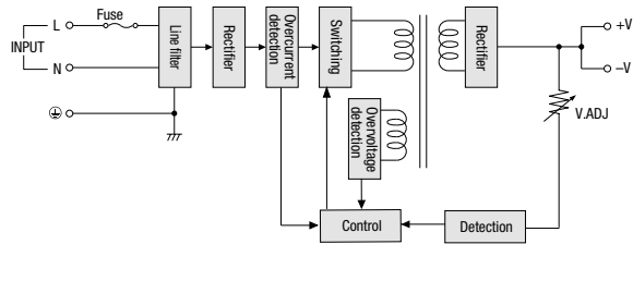
PS3V-030AF, PS3V-050AF
