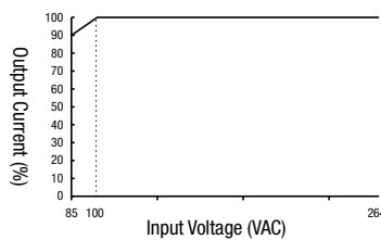
PS3V-050AF
