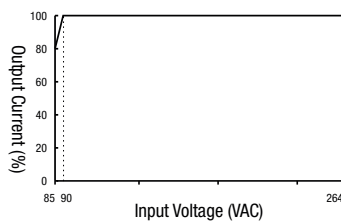
PS3V-015AF / -030AF
