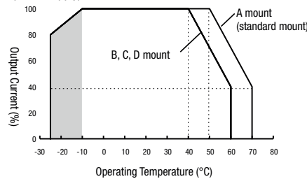
PS3V-015AF / -030AF
