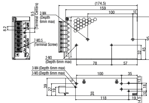
PS3V-150AF24C
