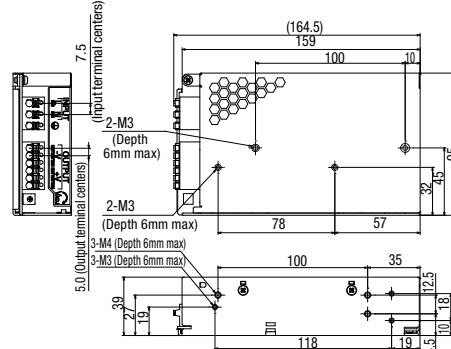
PS3V-150AF24P
