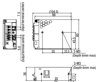
PS3V-150AF24P
