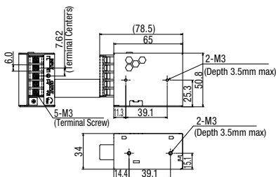
PS3V-015AF □ C
