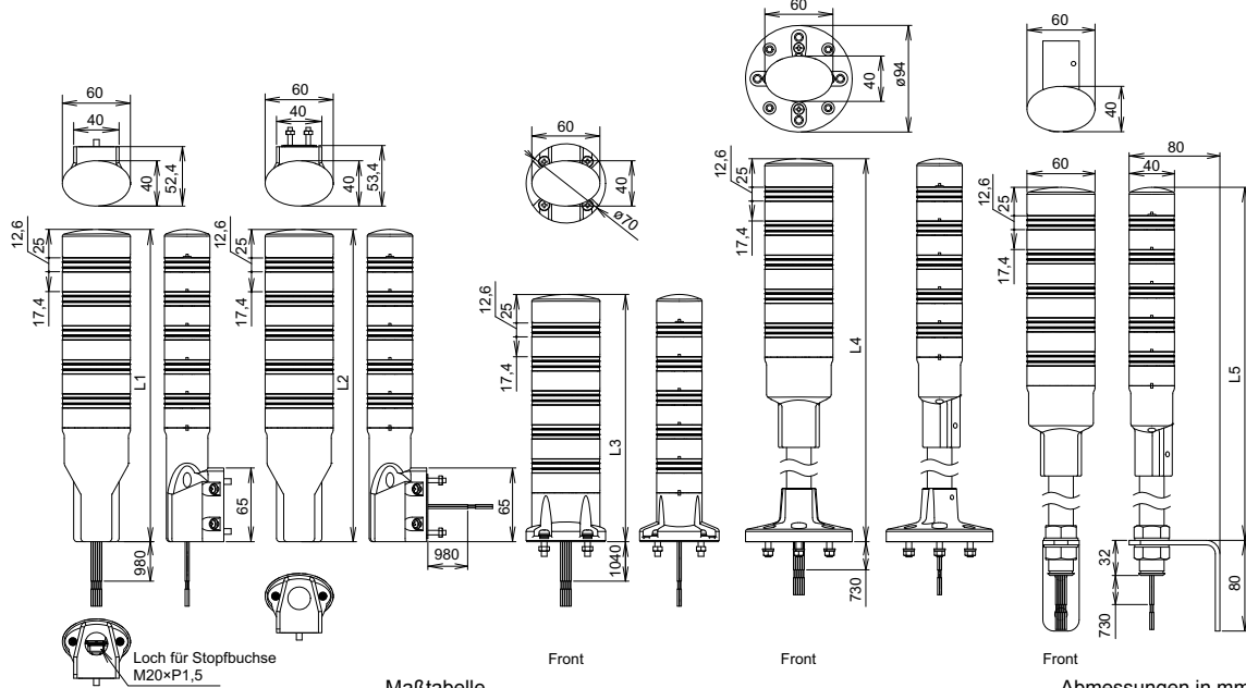
Maßtabelle
