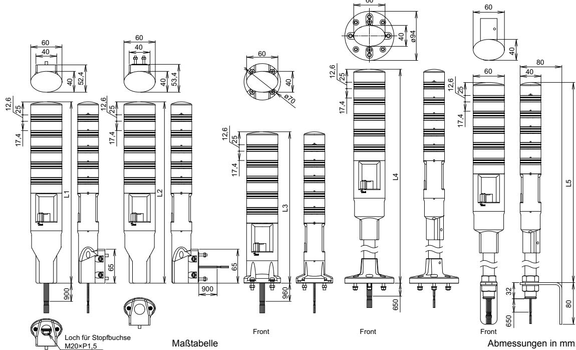
Maßtabelle
