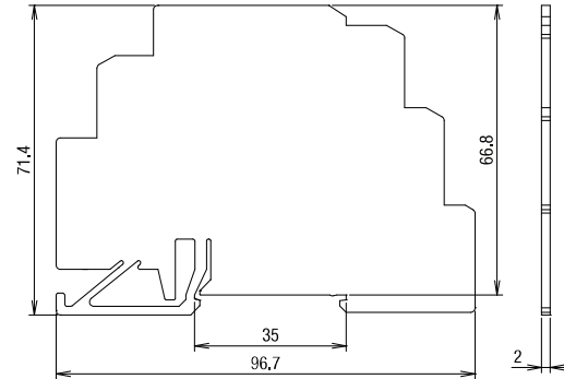
DIN Rail Spacer SV9Z-SA2W
