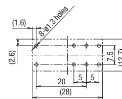
RF2V (DPDT)
