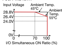
FC6A-M24BR1
